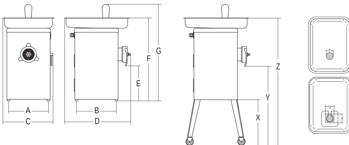
Gambe medie con ruote per TC 32 opzionali Optional medium legs with wheels for TC 32 x: 435 mm Y: 685 mm Z: 1005 mm
